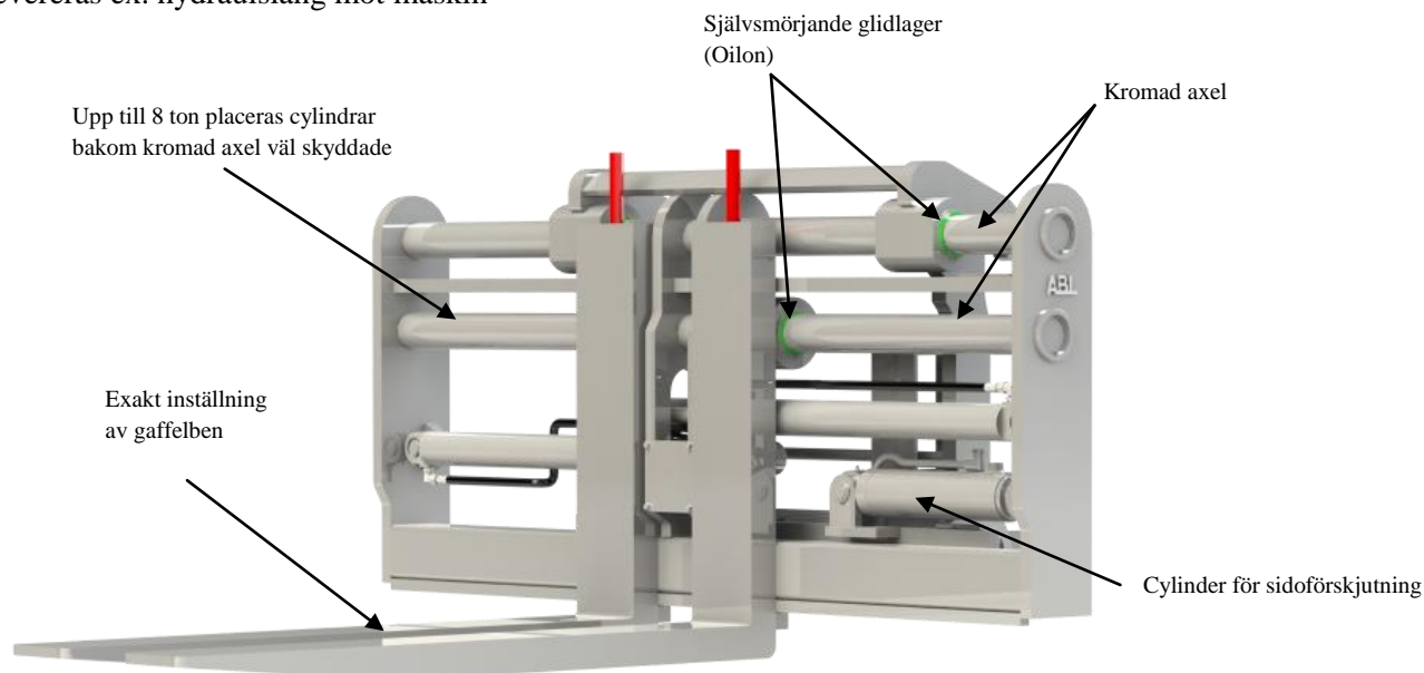
Bild 16T helhydraulisk pallgaffel
